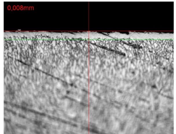
Abb. 4: Querschliff eines Expanite-gehärteten Bauteils aus Stellite 1040. Die Dicke der gehärteten Randzone liegt bei ca. 8µm, bei einer Oberflächenhärte von ca. 900HVO.025
