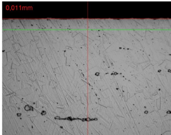
Abb. 3: Querschliff (Lichtmikroskopische Aufnahme) an einem Expanite-gehärteten Bauteil aus Inconel® 718 zeigt eine homogene Schichtdicke im Bereich von ca. 10µm. Oberflächenhärte-Messungen resultieren in Härtewerten von ca. 1.000 HVO.025
